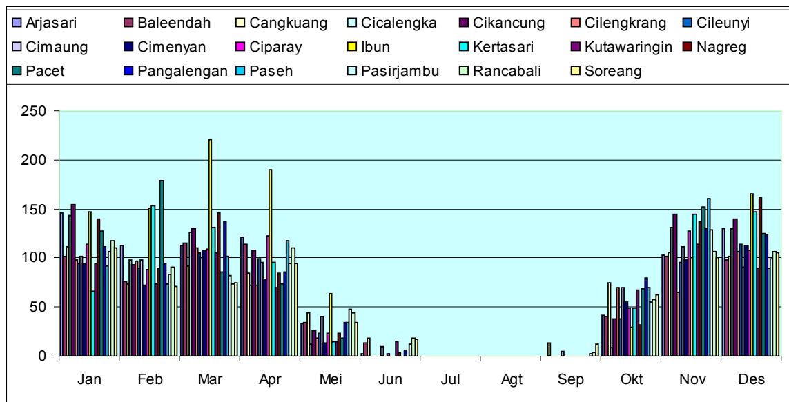
Gambar 3. Curah hujan efektif lokasi penelitian
