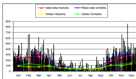
Gambar 2. Karakteristik curah hujan historis dan sintetis Kecamatan Pangalengan
