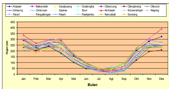
Gambar 1. Curah hujan wilayah rata-Rata Kabupaten Bandung
