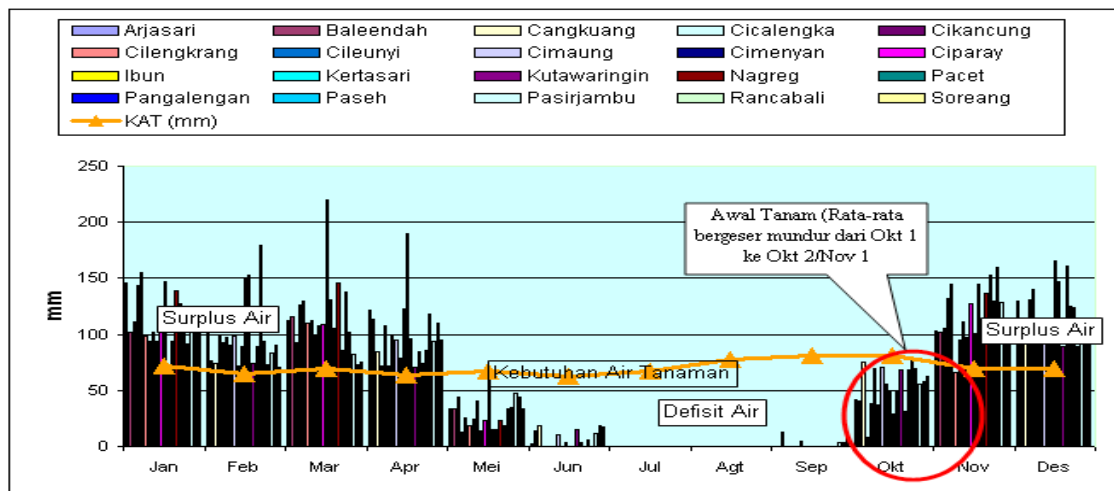
Gambar 5. Neraca Air Lahan Kering di Lokasi Penelitian
