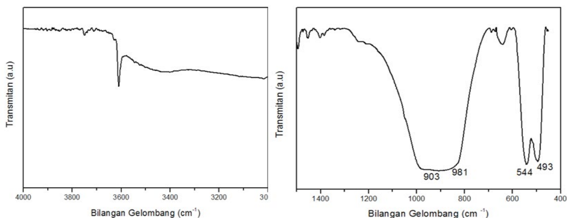
Gambar 3. Spektrum FTIR apatit hasil sintesis hidrotermal ( \text{La}_{9,33}\text{Si}_6\text{O}_{26} ) yang telah dipanaskan pada 120 °C.
