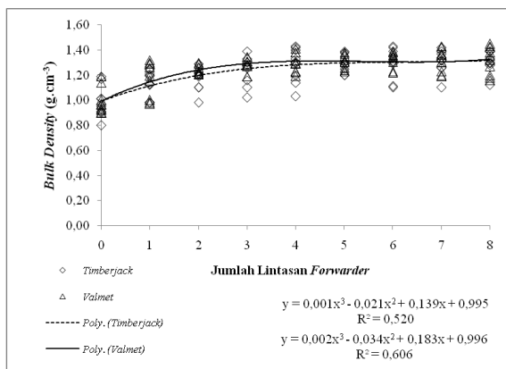
Gambar 2. Hubungan Bulk density terhadap jumlah lintasan forwarder Timberjack 1010b dan Valmet 860.1 .
