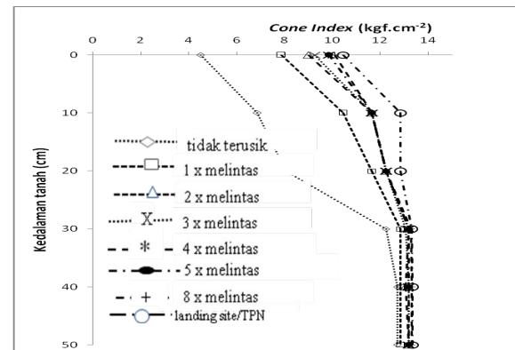
Gambar 4. Nilai cone index pada permukaan dan kedalaman tanah terhadap jumlah lintasan forwarder Valmet , tanah tidak terusik dan TPn
