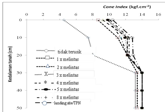
Gambar 3. Nilai cone index pada permukaan dan kedalaman tanah terhadap jumlah lintasan forwarder Timberjack , tanah tidak terusik dan pada TPn
