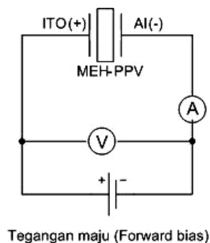
Gambar 2. Rangkaian untuk pengukuran karakteristik I-V
