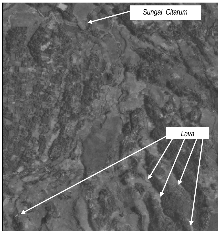
Gambar 3. Foto-udara bentangalam kawasan Malimping
