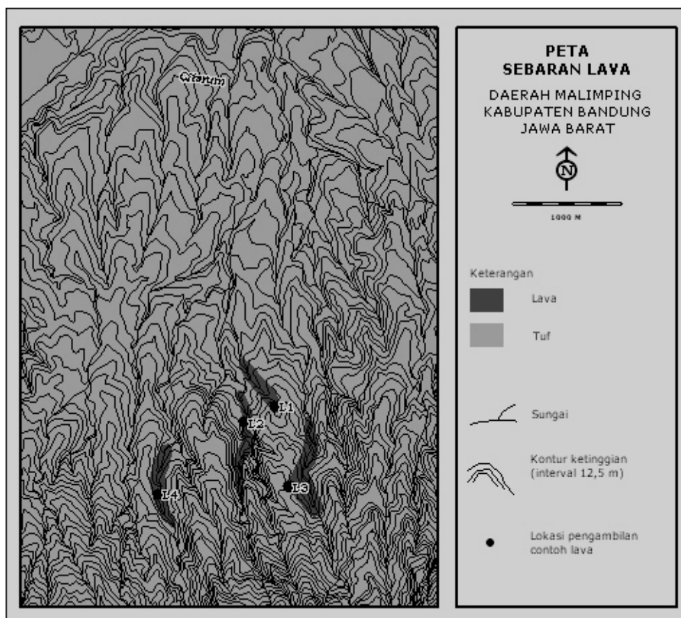
Gambar 5. Peta sebaran lava dan lokasi pengambilan sampel
